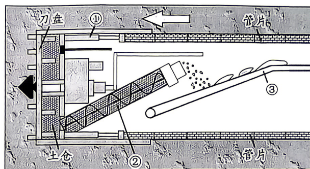
某盾构机内部结构剖面图
